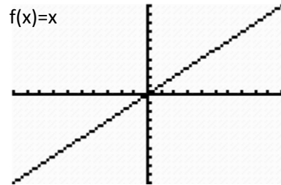
Linear Function
